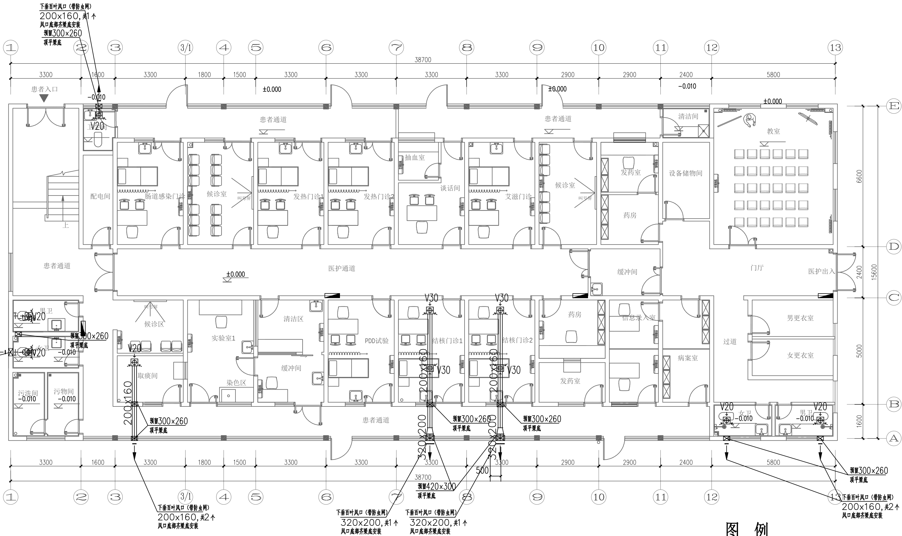
一层通风平面图 1:100
