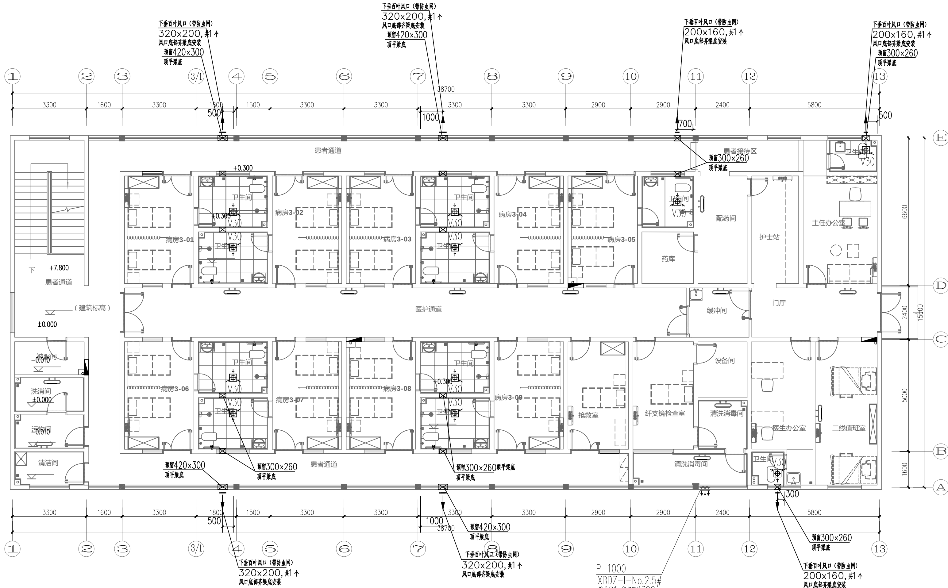
三层通风平面图 1:100
